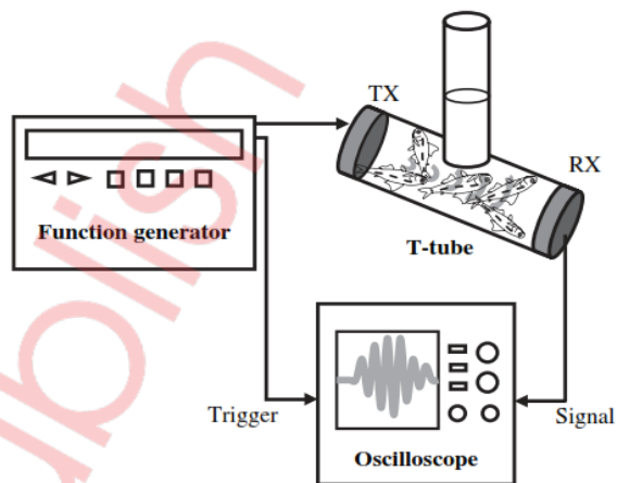
Gambar 3.3. Komponen dan Desain Pengukuran Kecepatan Suara Berdasarkan Teori pada Tahapan Mengukur Kekuatan Target Ikan Secara Teoretis (Yasuma et al. , 2006).
