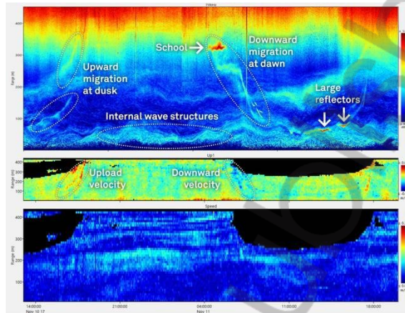
Gambar 4.17. Echogram (atas), Kecepatan Arus Vertikal (tengah), dan Kecepatan Arus secara Horizontal (bawah) (Gambar: Nortek; Laman: https://www.marinetechologynews.com ).
